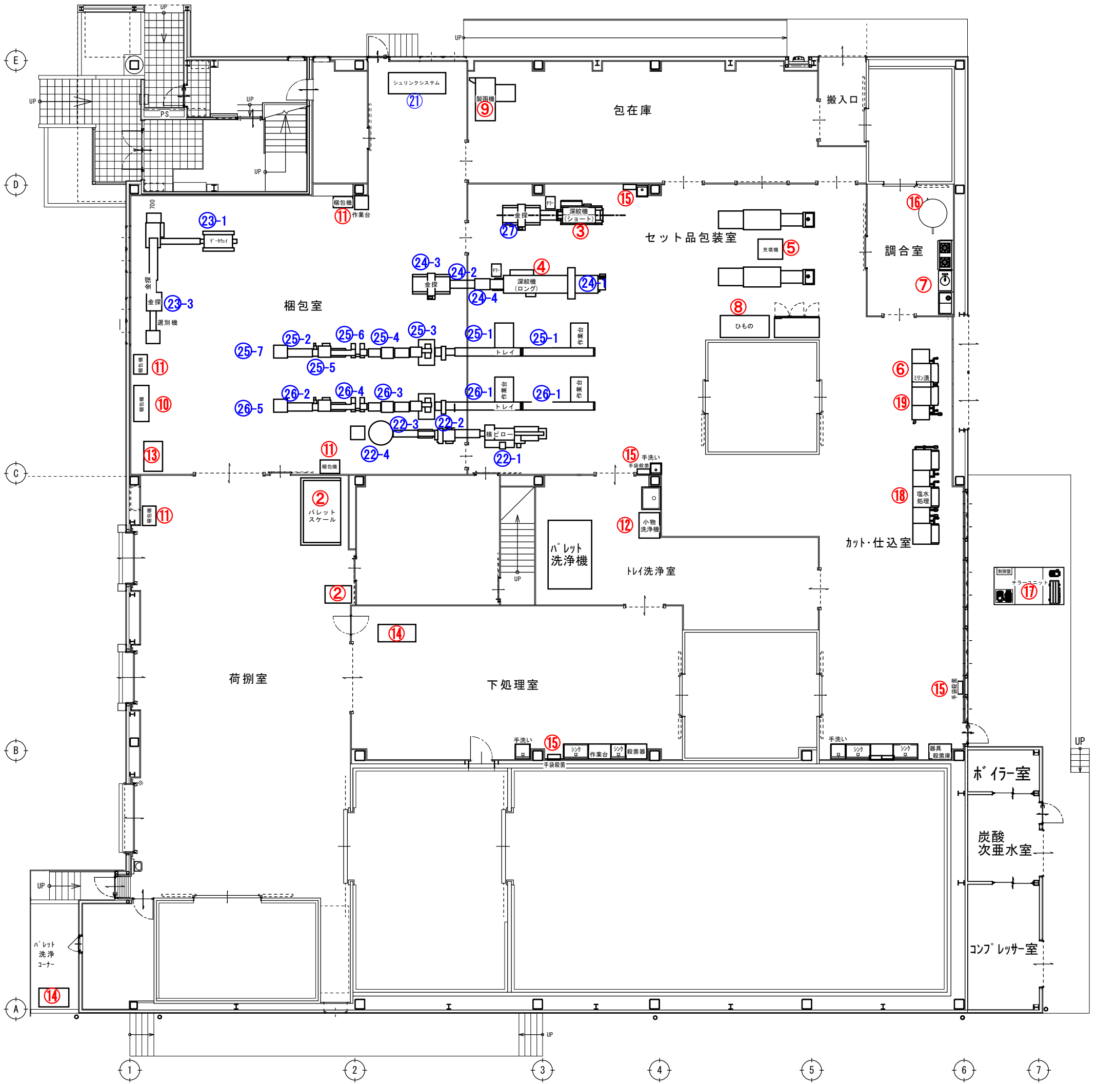
<補助対象機械レイアウト図>
